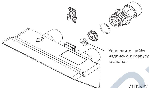
Рис. 5 - Ограничитель потока в дренажной линии диаметром 3/4 дюйма
