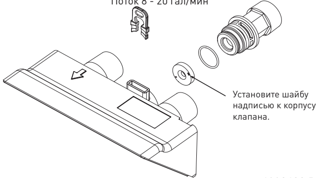
Рис. 4 - Ограничитель потока в дренажной линии диаметром 1 дюйм
